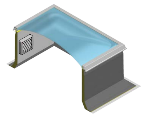
Elektroventilator Typ EV Ab Aufsatzkranzhöhe 300 mm: Entlüftungsventilator 150 m 3 /h, 230 V/50 Hz. Zusätzlich ab Aufsatzkranzhöhe 40 cm: Be- und Entlüftungsventilatoren mit 500 m 3 /h oder 1.000 m 3 /h, 230 V/50 Hz
